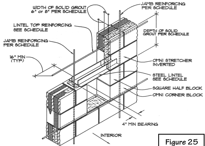
○ WINDOW / DOOR JAMB DETAIL
